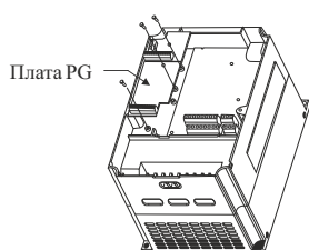
Способ установки платы расширения PG
