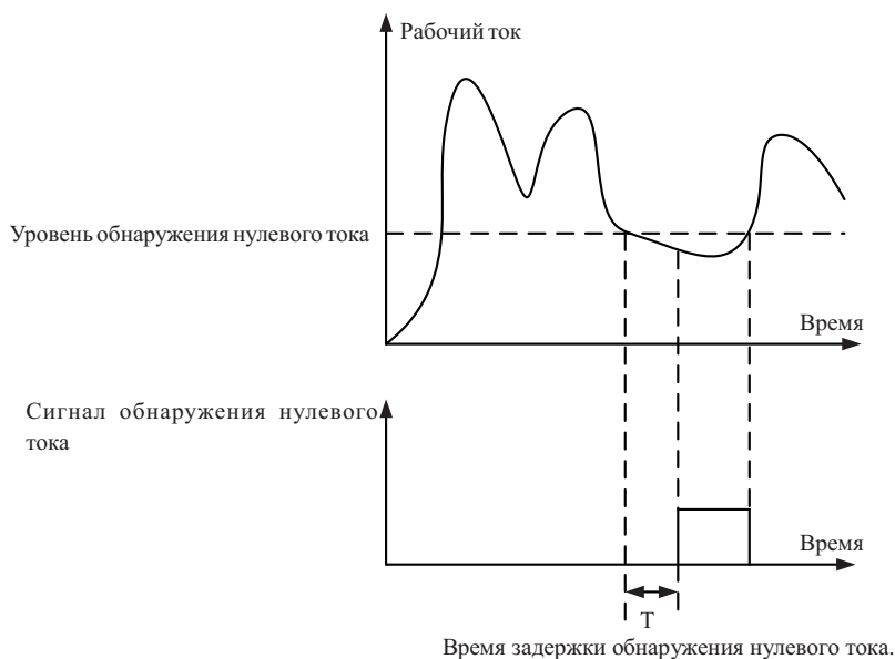
Время задержки обнаружения нулевого тока.
