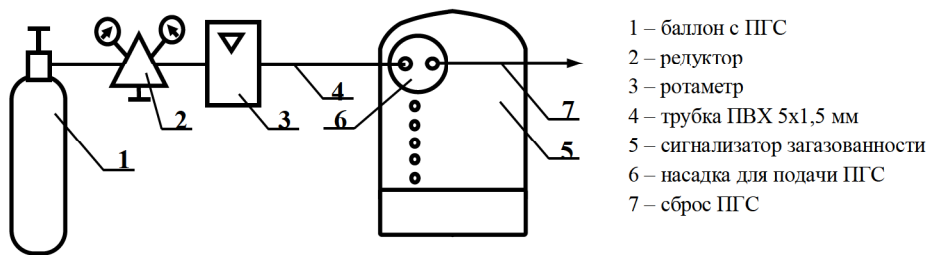
Рисунок Д.1 – Схема для настройки порогов срабатывания
