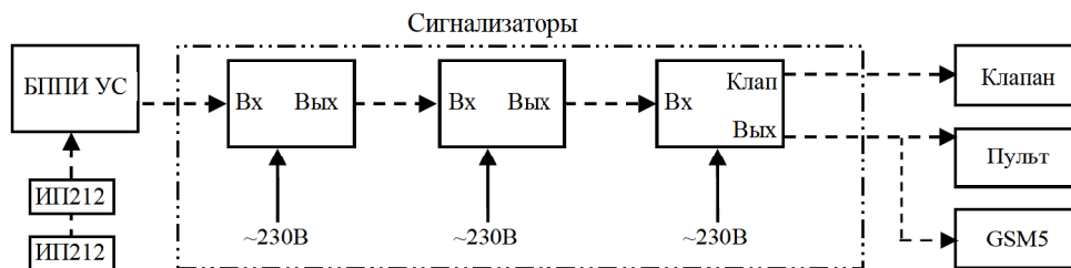
Рисунок 1 – Структурная схема
