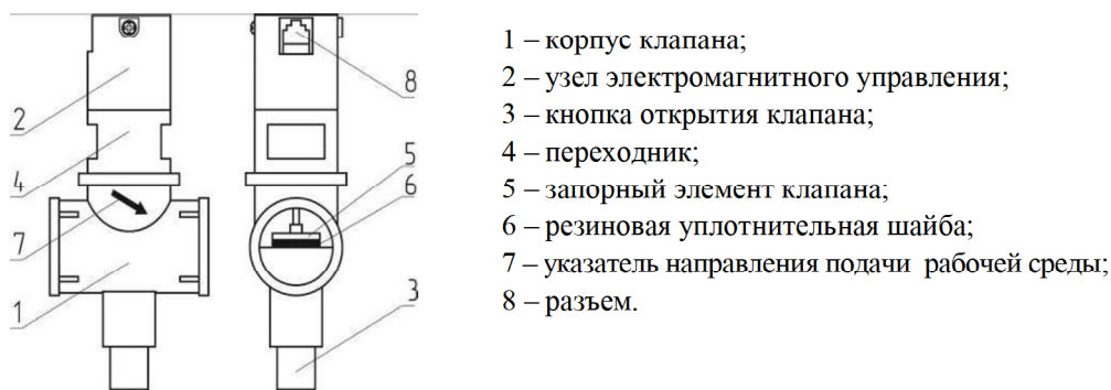
Рисунок 3 – Внешний вид клапана КЗЭУГ.
