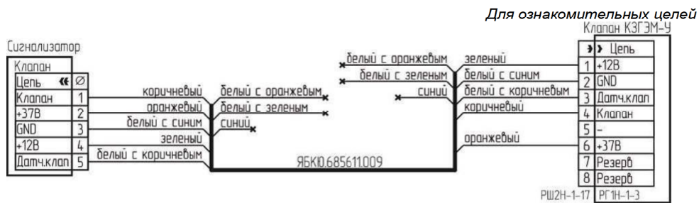
Рисунок Б.3 – Схема подключения клапана КЗГЭМ-У с разъемом РГ1Н-1-3.
