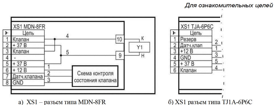
Рисунок 4 – Клапан КЗЭУГ. Схема электрическая принципиальная.
