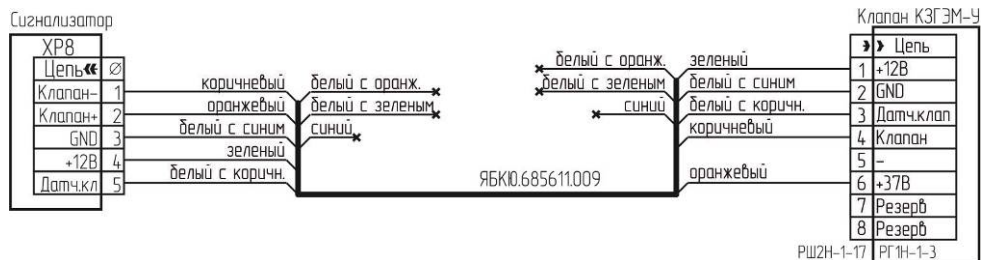
Рисунок Г.5 – Схема подключения клапана КЗГЭМ-У с разъемом РГ1Н-1-3.
