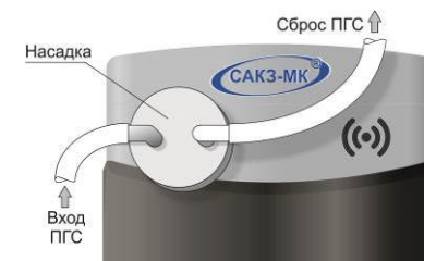
Рисунок Д.1 – Схема установки насадки
