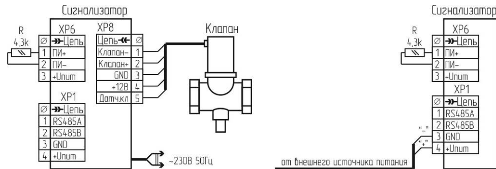
Рисунок Г.1 – Типовая схема подключения клапана (кроме СЗ-3ЕВ)
