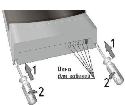
Рисунок В.2 – Снятие клеммной крышки
