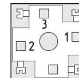
Вилка на кабель PSH2H-1-17, нумерация контактов (вид со стороны пайки)
