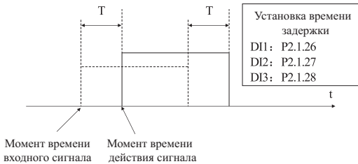
T - время задержки сигнала
