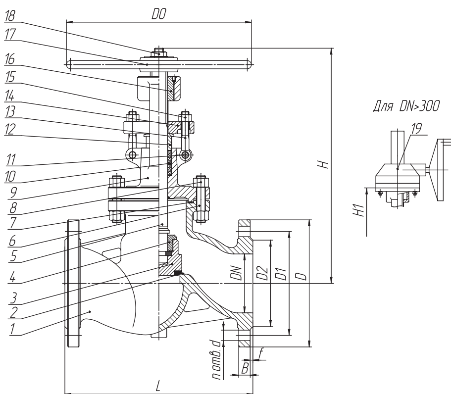
Рис. 2.2 — Клапан запорный PN 2,5 МПа
