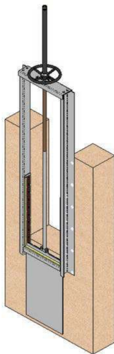
Маховик с выдвижным штоком
