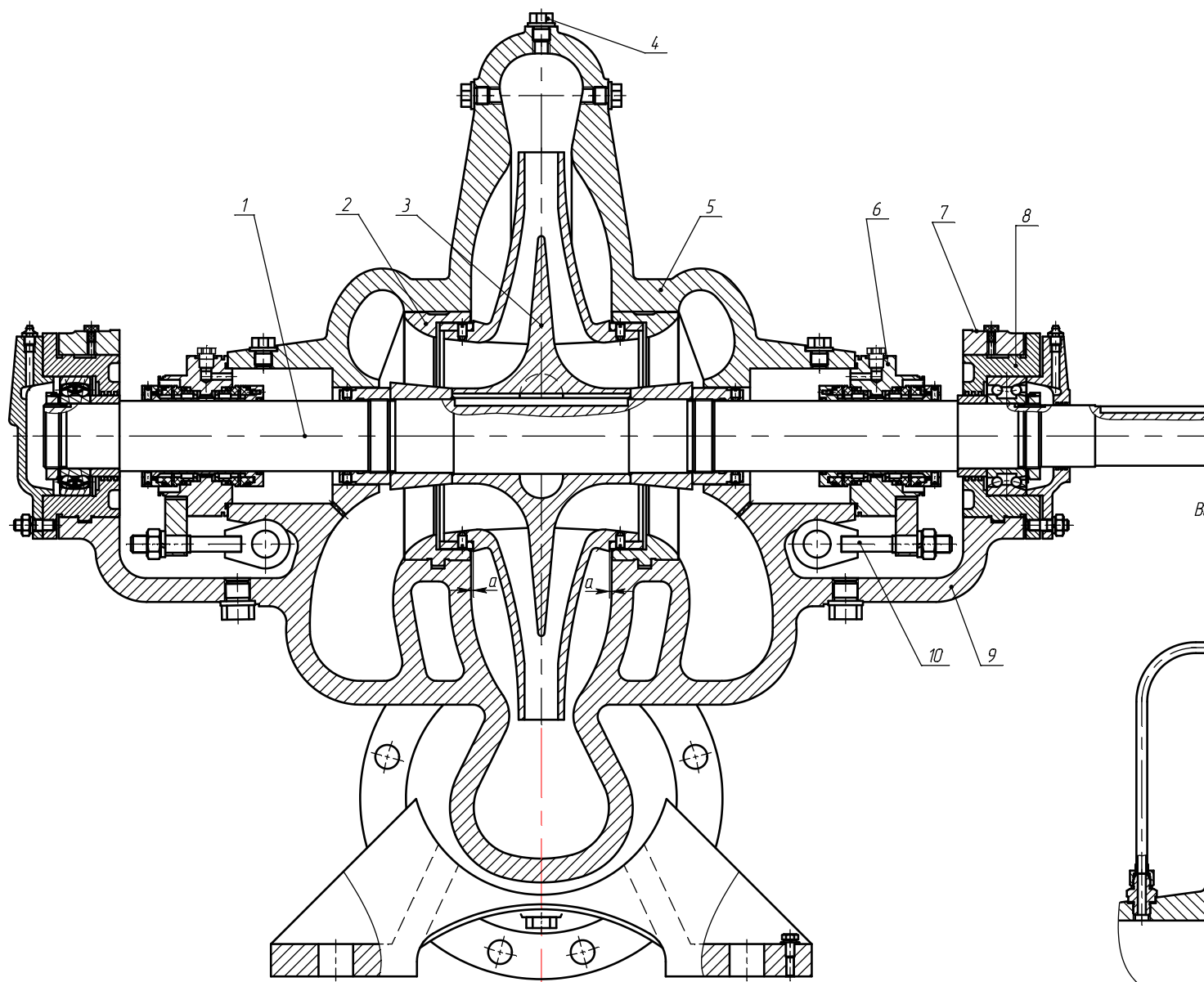
Рисунок 1 – Разрез насоса
