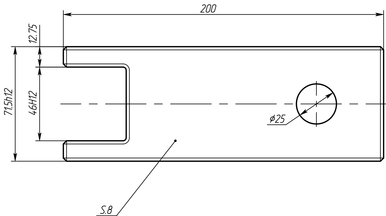
Рисунок 4. Ключ шлицевый
