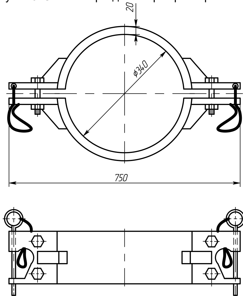
Рисунок 7. Хомут монтажный.
