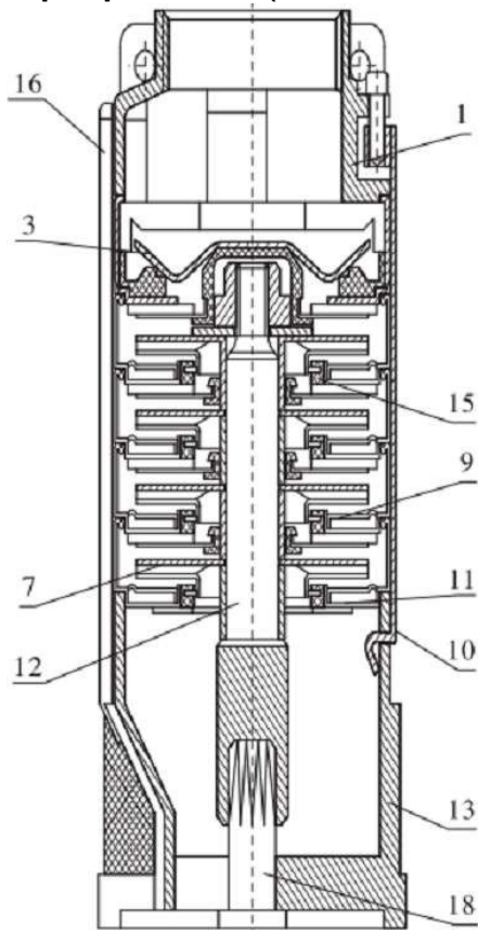
Вид в разрезе SJ5 (насосная часть)
