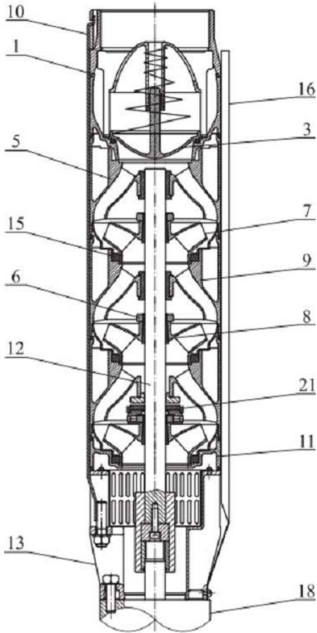
Вид в разрезе SJ95 (насосная часть)
