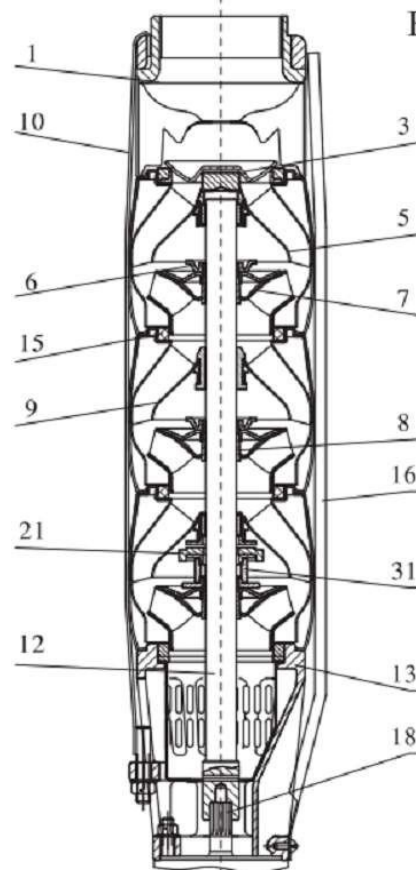
Вид в разрезе SJ42 (насосная часть)
